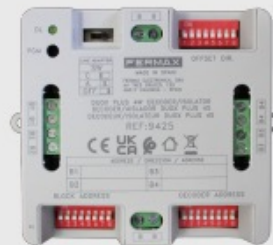
9425 DUOX PLUS 4-OUT DECODER ISOLATORE
